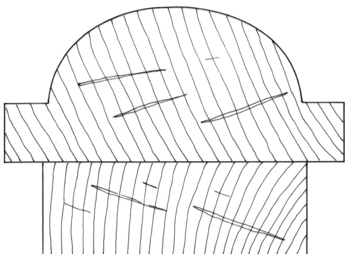
B / Profil du meneau 2 éléments cloués (échelle 1)
