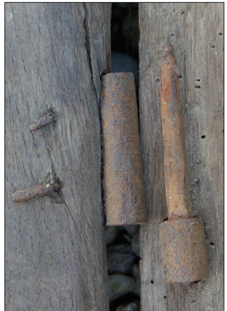
Fig. 1.5. Fiche à gond
