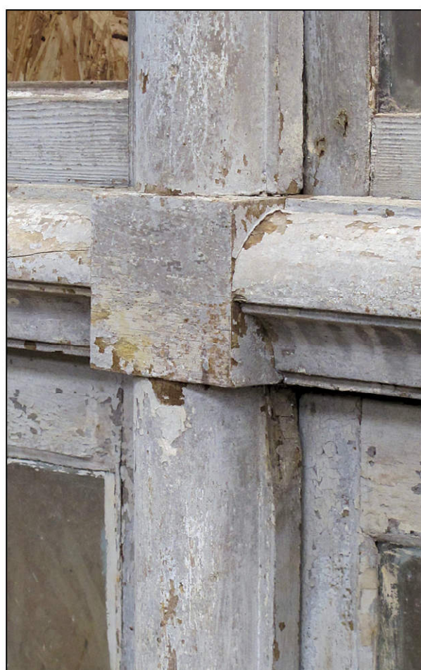
Fig. 3.3. Assemblage meneau / croisillon
