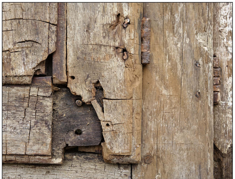
Fig. 3.4. Volet inférieur (assemblage) et fiches
