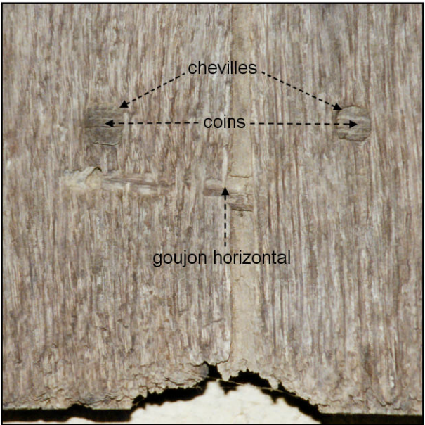
Fig. 3.6. Assemblage du volet (détail)
