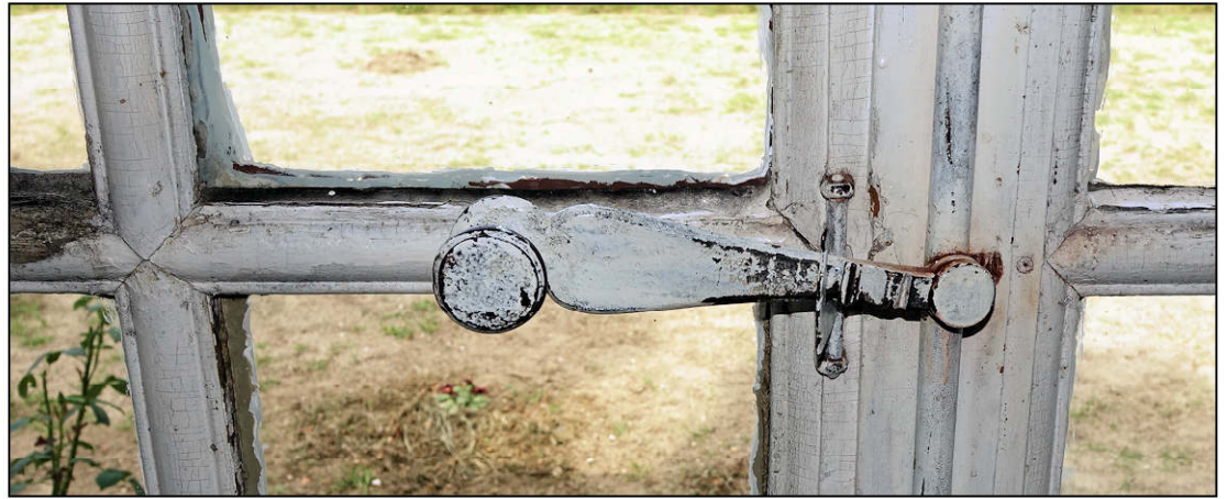
Fig. 9.2. Espagnolette (poignée et arrêtoir à charnière)
