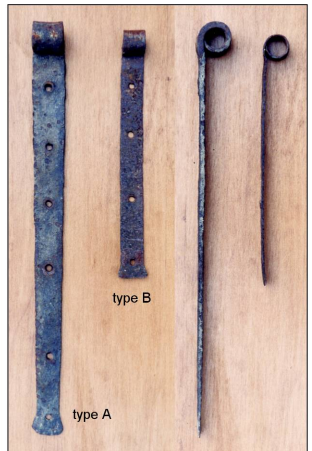
Fig. 1.6. Pentures
