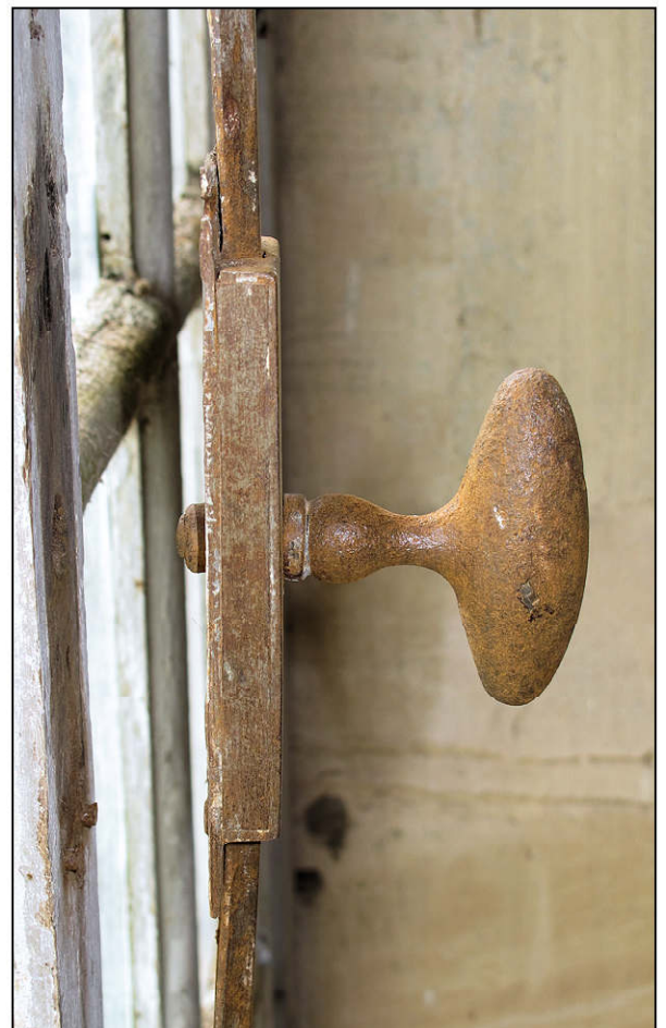
Fig. 11.7. Crémone / boîte et poignée
