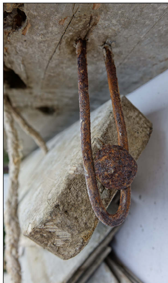
Fig. 6.7. Agrafe et tourillon (côté droit)
